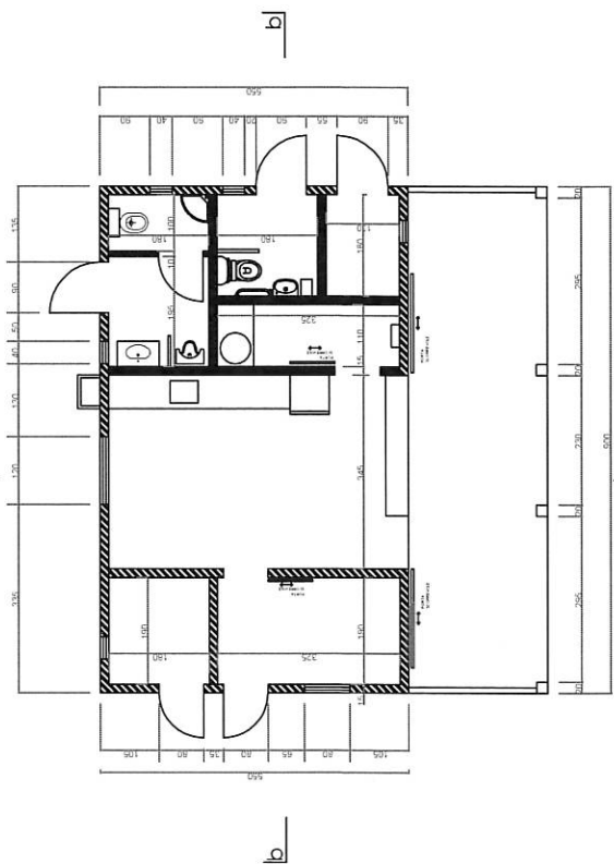
pianta
